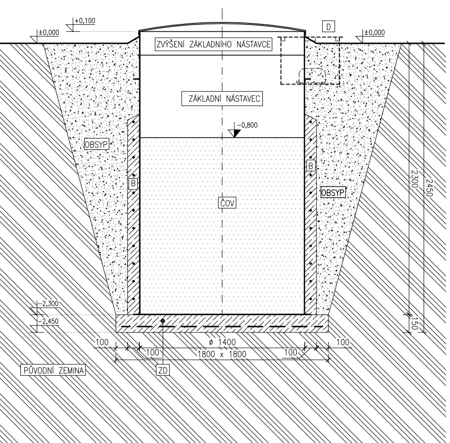
Řez
